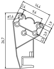
Piastra per travetti in legno SK 2500-5 in acciaio
