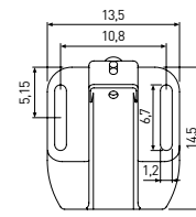
Piastra inclinata a soffitto SK 2500-4 in acciaio
