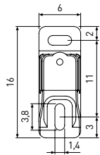
Piastra stretta SK 2500-2 in acciaio a parete
