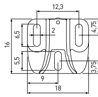
Piastra per cappotto SK 2500 037 in alluminio
