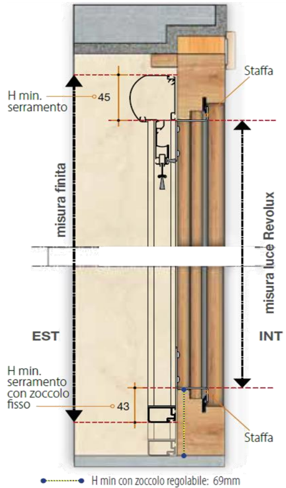
Sezione orizzontale
