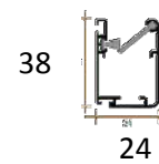
Guida antivento
