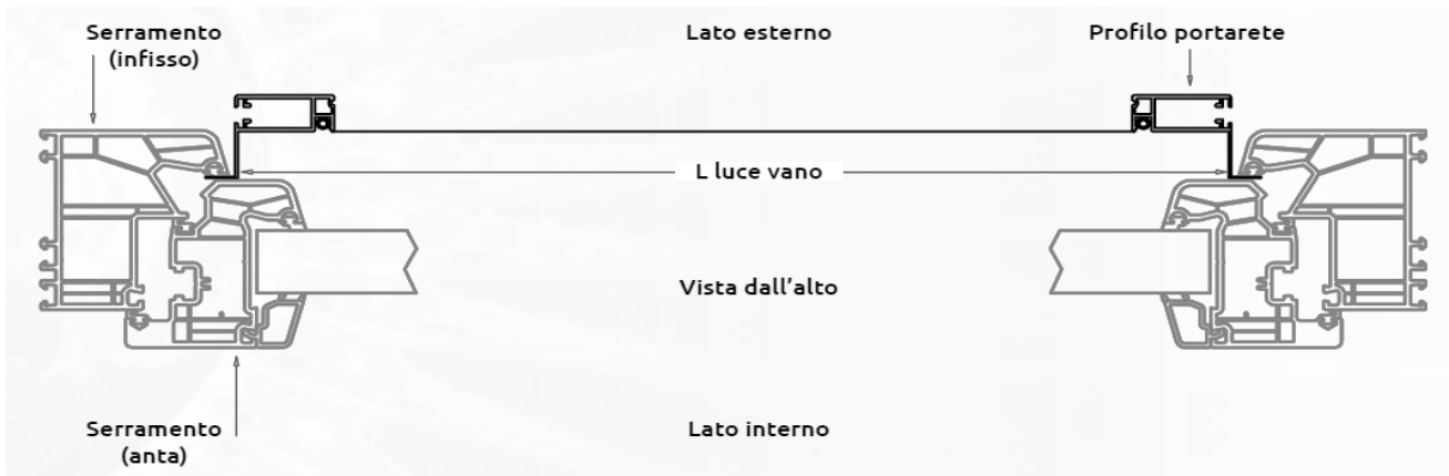
Sezione orizzontale
